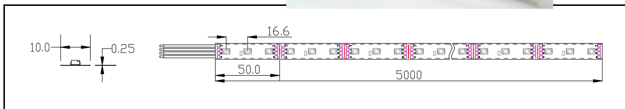
Måttbeskrivning (mm)
